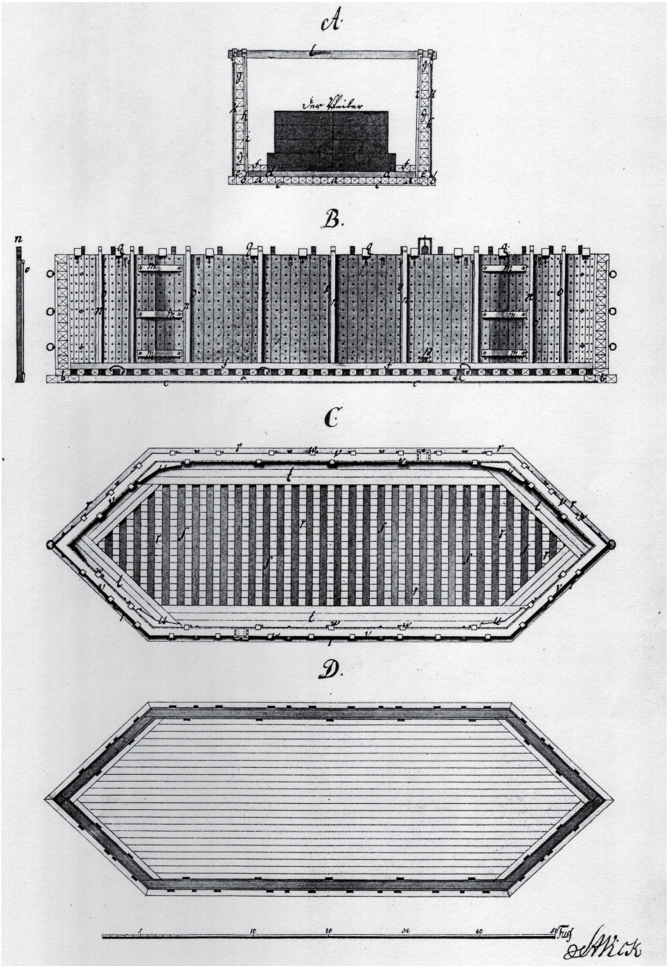
8 | „Profil eines Kastens worin die Pfeiler zu der Brücke so zu London neu gebaut wird gemauert und auf den Grund gesetzt werden“, Bestandsplan eines Senkkastens zur Gründung der Westminster Bridge von Charles Labelye, lavierte Tuschezeichnung, Sudfeld Andreas Vick, um 1744 (Hardenbergsches Familienarchiv Nr. 1525, fol. 36).
