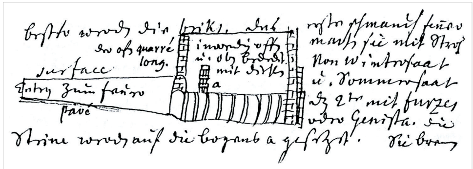
[Schnittzeichnung eines Ziegelbrennofens in Holkham Hall: der Ofen quarré long. inwendig offen u.[nd] oben bedeckt mit Diehlen [-] surface [-] Entry [-] zum Feuer pavé]
